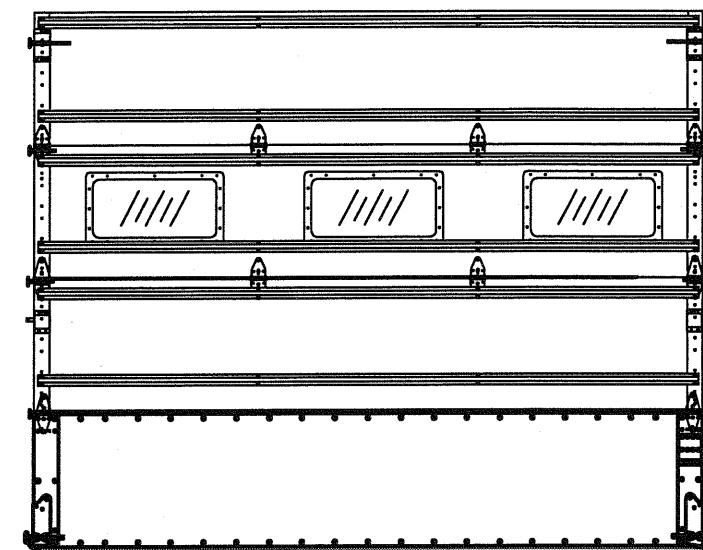
OPTIONAL SINGLE SUPERFLEX SECTION N.T.S.
