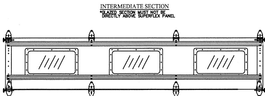
OPTIONAL GLAZED SECTION W/ 24" X 12" WINDOWS N.T.S.
